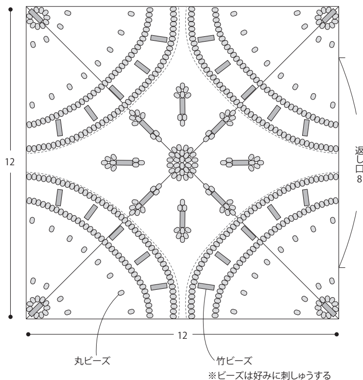
配置図
